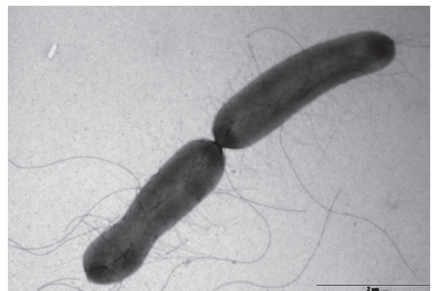
Mikroskopaufnahme von zwei E. coli -Bakterien (© Dr. Jochen Reetz, BfR)
